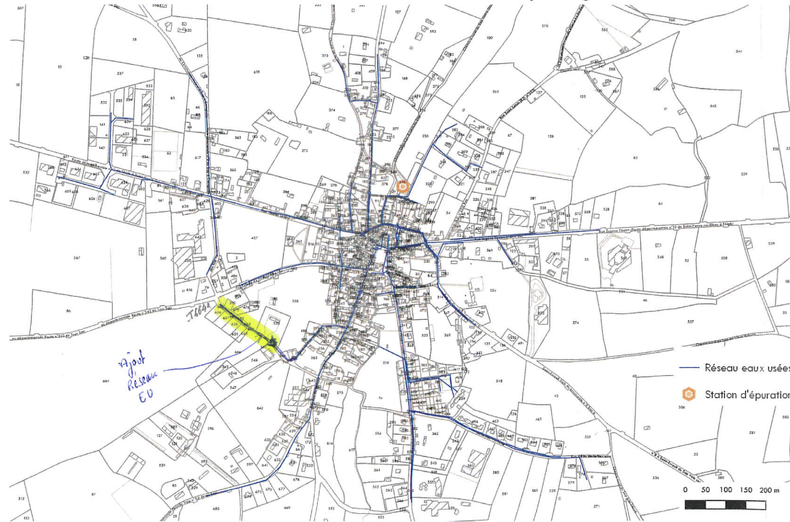
Plan du réseau des eaux usées - Commune du Sap en Auge
